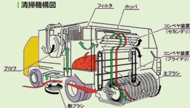
清掃機構図
