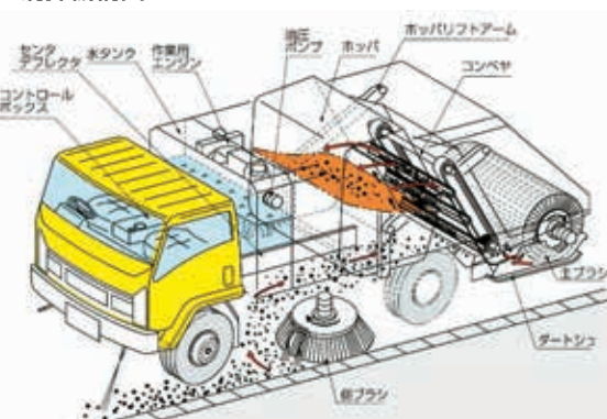
清掃機構図
