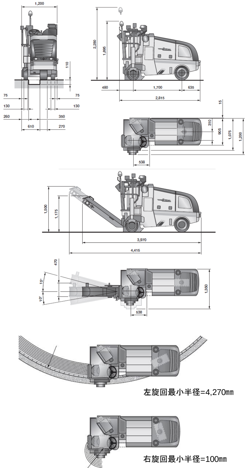
機械寸法(単位:mm)
